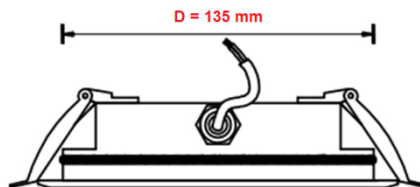
Montage in der Decke
