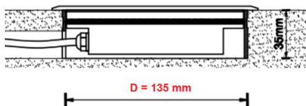
Montage im Boden
