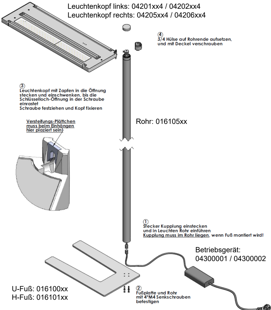
Abb. Montage
